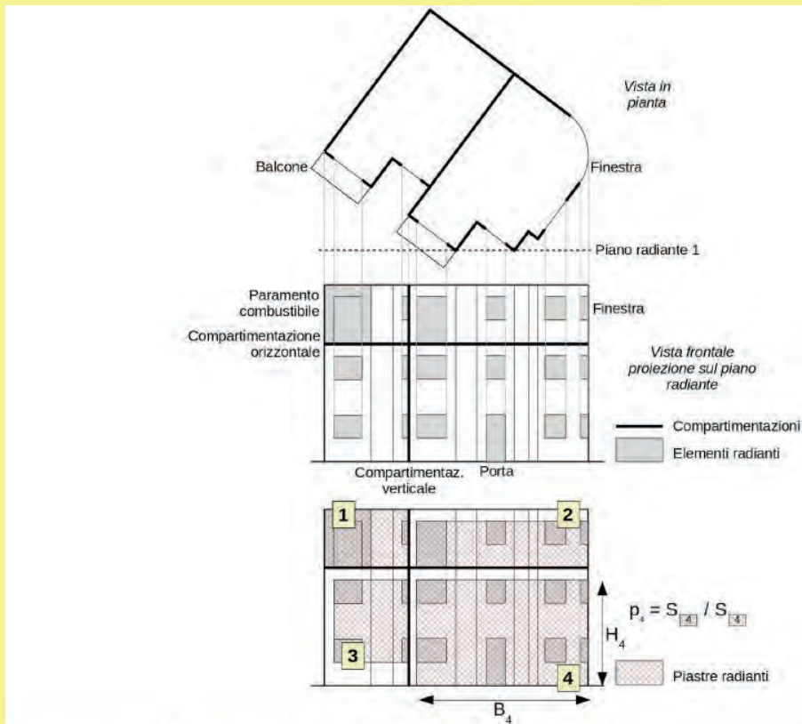
Illustrazione S.3-2: Determinazione delle piastreradianti, vista in pianta e frontale
